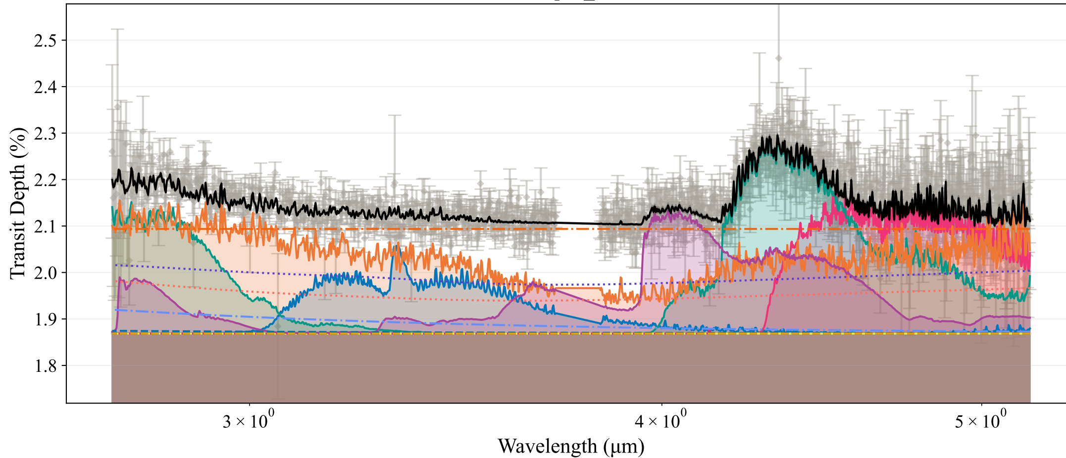
nirspec_iso
